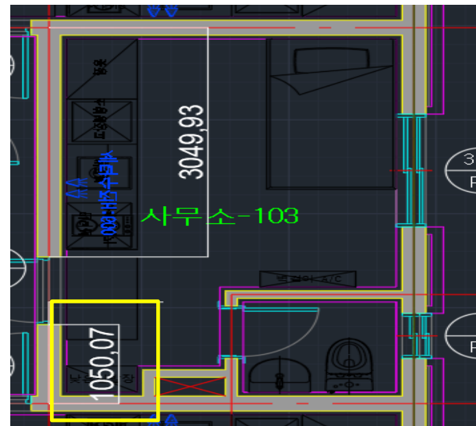
시공도면
